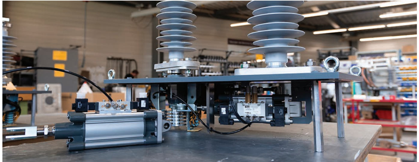
Montage du disjoncteur équipé du distributeur Parker Viking : composants robustes et résistants aux intempéries, destinés à l'industrie ferroviaire de production.
