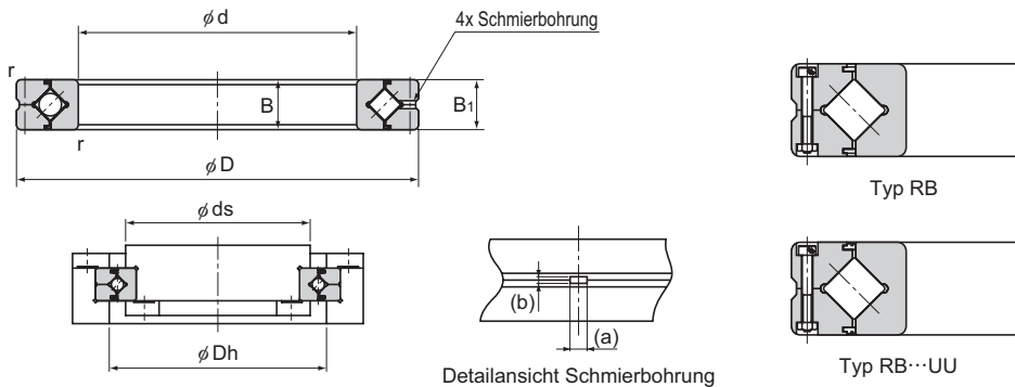
Detailansicht Schmierbohrung
