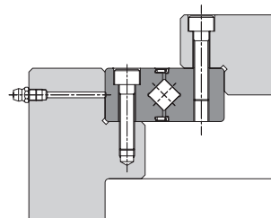
Montagebeispiel RU - 2
